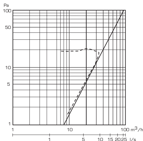
Kapacitet uppmätt tillsammans med Fresh 100.
