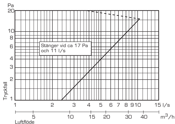
Kapacitet uppmätt tillsammans med TL98P.
