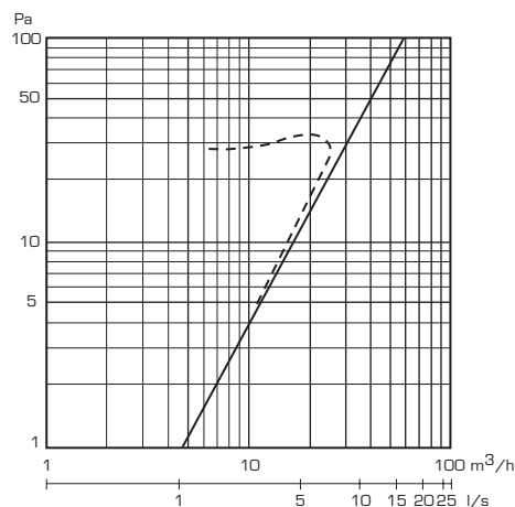
Kapacitet uppmätt tillsammans med Fresh 80.
